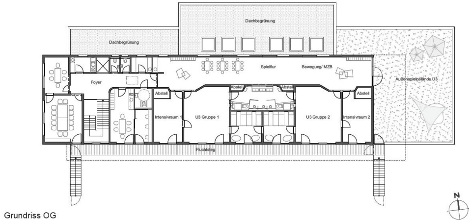
Grundriss OG
